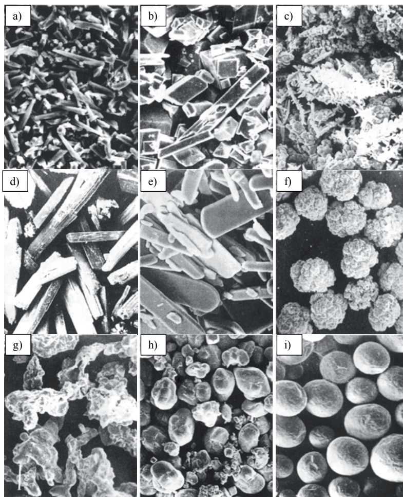
Ryc. 1. Kształt cząstek proszków: a) iglasty, b) wielościenny, c) dendrytyczny, d) włóknisty, e) płatkowy, f) granulowy, g) nieregularny, h) globularny, i) kulisty [9] Fig. 1. Particle shape of powders: a) needle shaped, b) polyhedral, c) dendritic, d) fibrous, e) patch, f) granular, g) irregular, h) globular, i) spherical [9]
