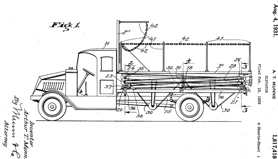
Ryc. 5. Opatentowana konstrukcja windy na podwoziu samojezdnym autorstwa Artura T. Munnsa [5]. Fig. 5. Construction of the elevator on the self-propelled chassis patented by Arthur T. Munns [5].
